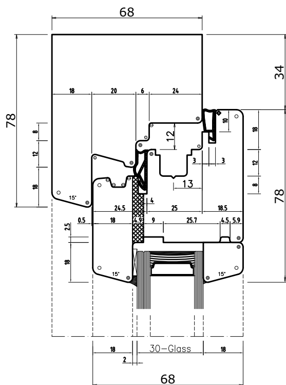
Sectiune verticala
