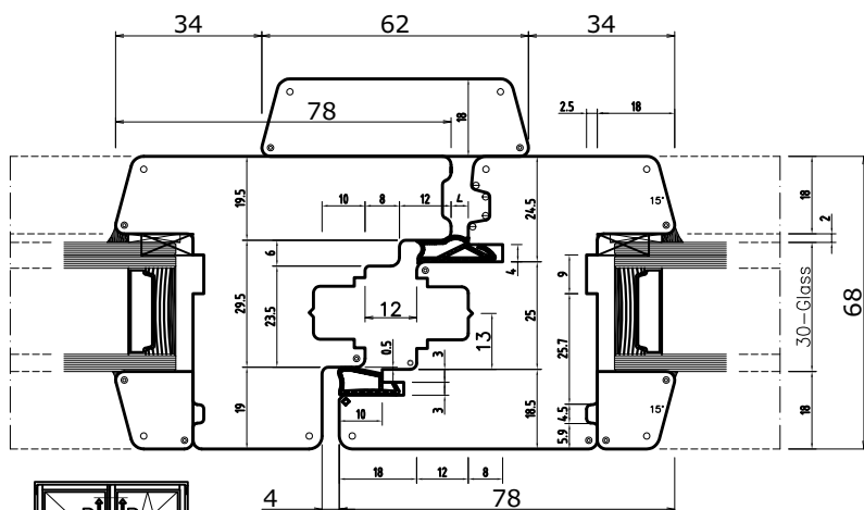
Sectiune verticala
